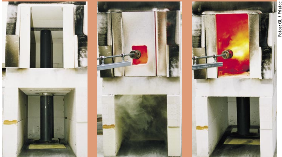
Bild 2 Orientierender Brandversuch von Friatec. Links: Friaphon-Rohr mit Brandschutzmanschette entsprechend Zulassung. Mitte: Über 1000°C in der oberen Kammer. Rechts: Nach über 90 Minuten kein Durchbrand nach unten. Die Brandschutzmanschette in der unteren Kammer schloss nur unvollständig. Eine Brandausbreitung nach unten erfolgte nicht, brennendes Abtropfen/Abfallen trat nicht auf
